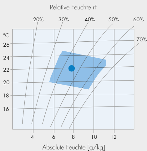
hx-Diagramm mit Darstellung des Bereichs der Komfortzone und des Arbeitspunkts
