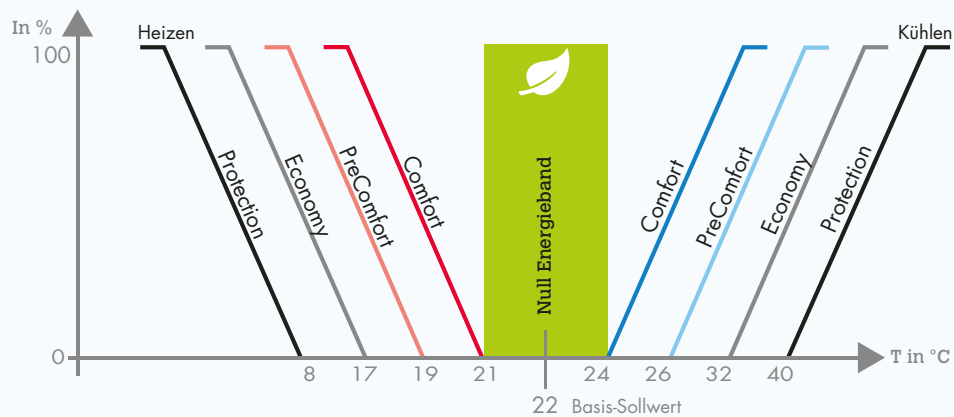
Grafik Sollwerte für verschiedene Energieniveaus (Quelle: VDI 3813)
